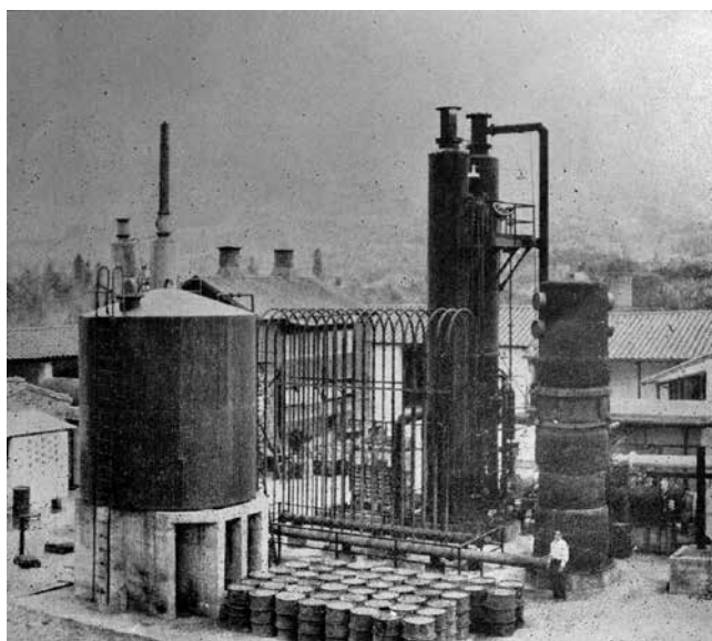
Figura 4. Anónimo, enero de 1951, "Vistas parciales de la planta de ácido sulfúrico" (fotografía en la revista Química e Industria , Biblioteca Nacional de Colombia, Hemeroteca Manuel del Socorro Rodríguez, Bogotá, 32).
