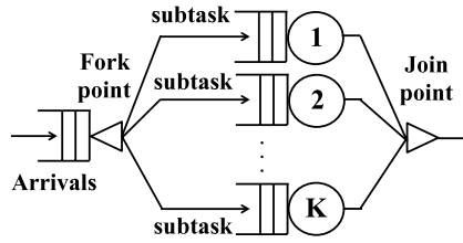
Fig. 1. Fork-join queue.
