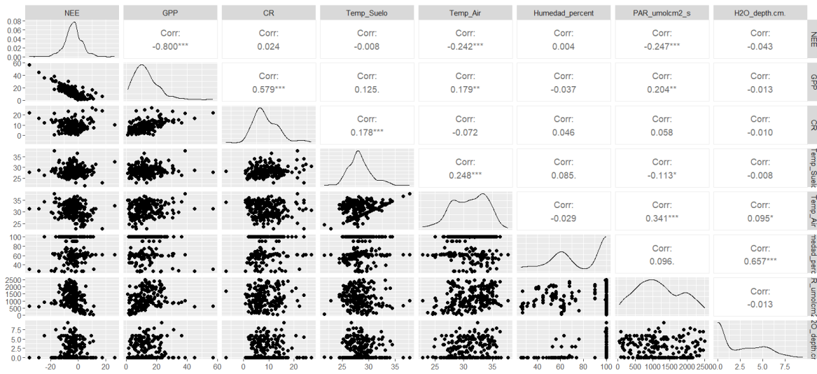
Figura S2. Correlación entre variables numéricas para evaluar relación y futura construcción de modelos.
