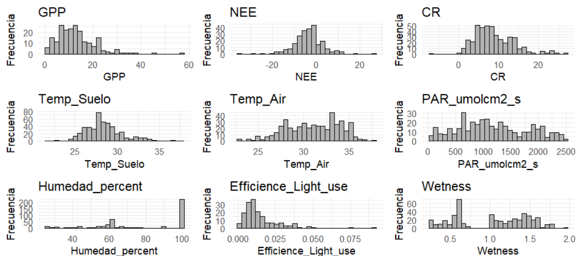
Figura S1. Histograma de variables numéricas. Distribución de las variables numéricas para el estudio preliminar de los datos.
